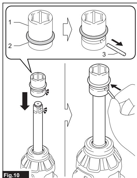
► 1. Douille à choc 2. Joint torique 3. Broche
